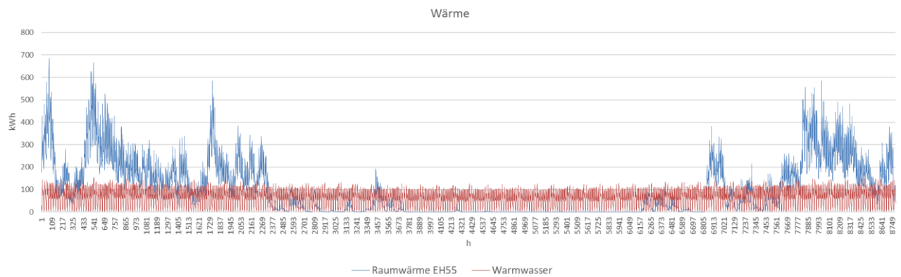
Abbildung 1 Lastprofil Warmwasser und Raumwärme für EH55-Standard
